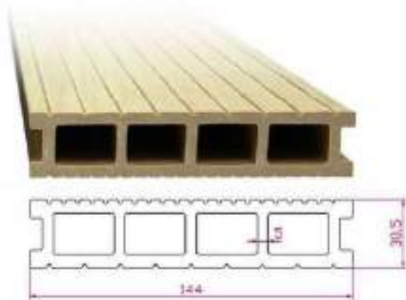
Илл. 1.1.12. ПУСТОТНАЯ КОМПОЗИТНАЯ ТЕРРАСНАЯ ДОСКА
