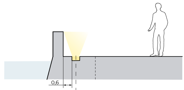
Светильник, встроенный в покрытие береговой зоны
