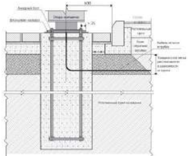
Илл. 4.1.11. КРЕПЛЕНИЕ ОПОРЫ ОСВЕЩЕНИЯ НА АНКЕРНЫХ ЗАКЛАДНЫХ
