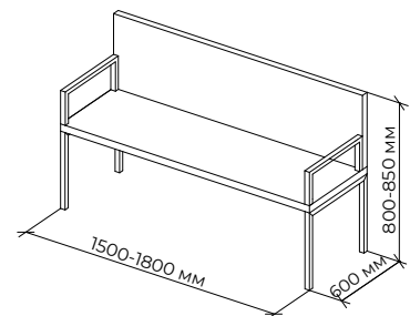
Скамья с подлокотниками
